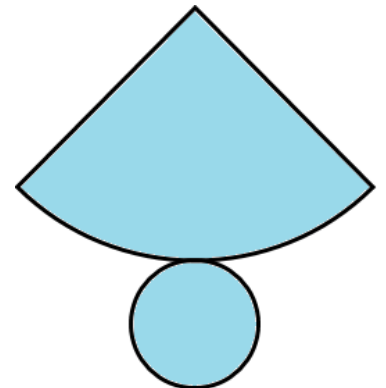
Cone
